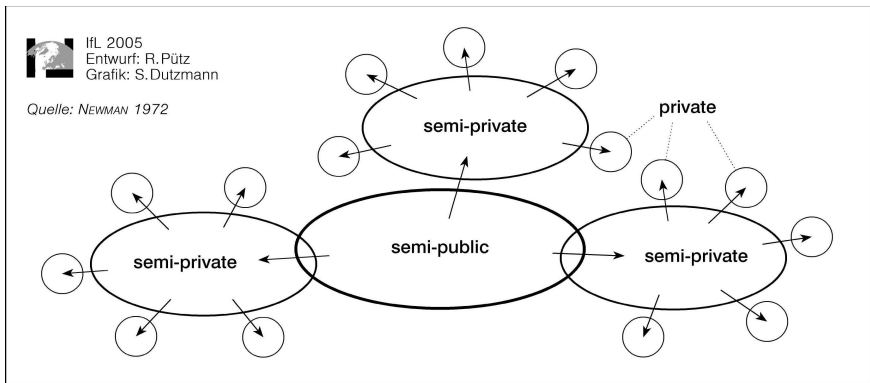
Abb. 2: Schema Oscar NEWMANs Zonierung der Wohnumwelt im Konzept des „defensible space“ (1972)
